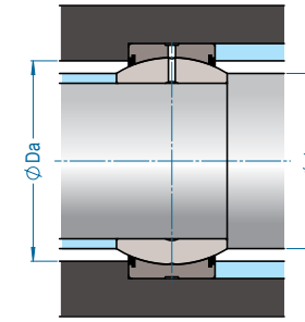
GE(00)FO 2RS dimensões de montagem
